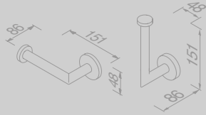
Toiletrolhouder / Reserverolhouder Toilet roll holder / Spare toilet roll holder 916509-02
