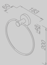
Handdoekkring Towel ring 916504-05
