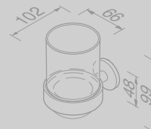
Glashouder met glas Glass holder with glass
