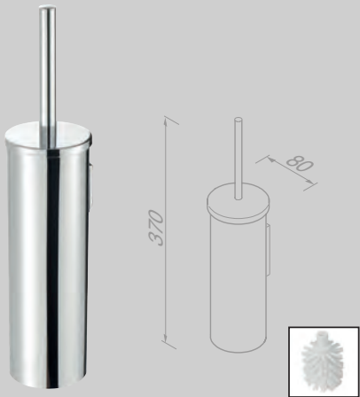
Toiletborstel met houder muurbevestiging Toilet brush and holder wall-mounted 916511-02
