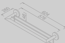
Handdoekrek met planchet 60 cm Towel rail with shelf 60 cm
