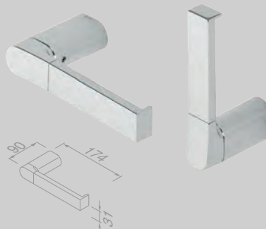
Toiletrolhouder / Reserverolhouder Toilet roll holder / Spare toilet roll holder 914509-02
