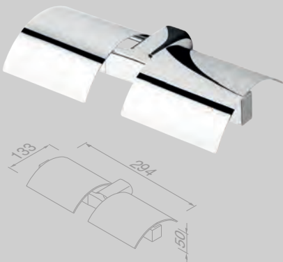
Toiletrolhouder met klep dubbel Toilet roll holder with cover double 914519-02
