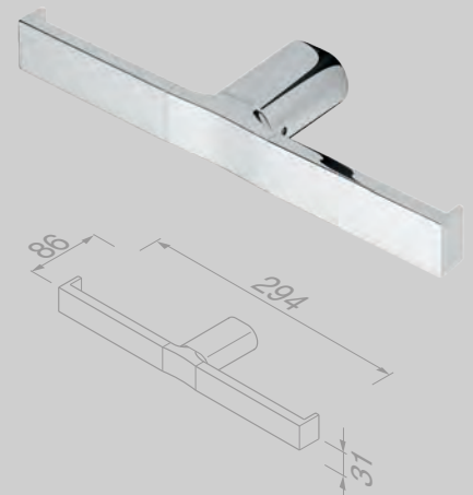
Toiletrolhouder dubbel Toilet roll holder double 914518-02
